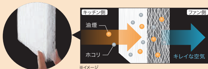
■ダスキンレンジフードフィルター(ガラス繊維タイプ)断面図
